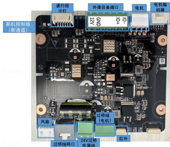
图5-8 副机控制板端口介绍
