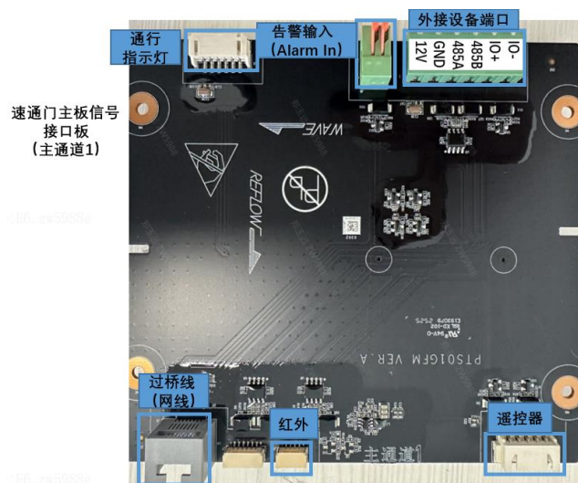
图5-7 主通道板端口介绍
