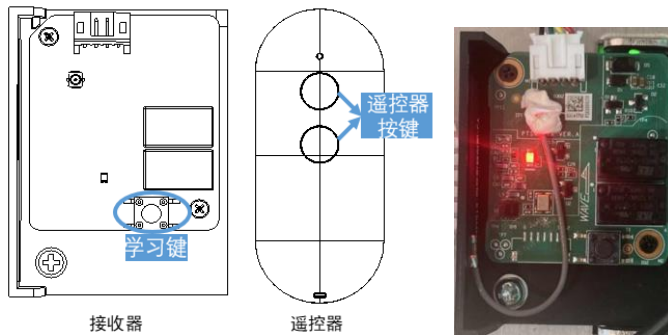
图5-18 接收器和遥控器简介图
