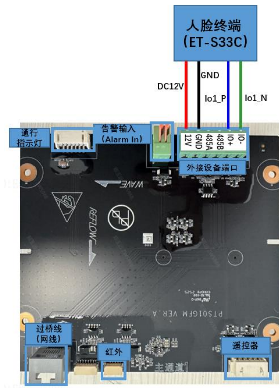
图5-10 人脸核验终端接线
