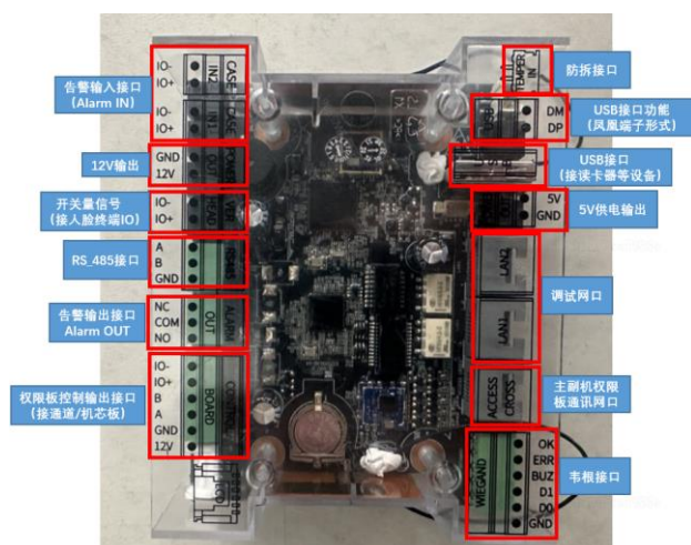
图5-13 权限板端口介绍
