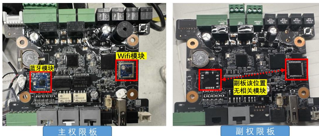
图5-13 权限板端口介绍
