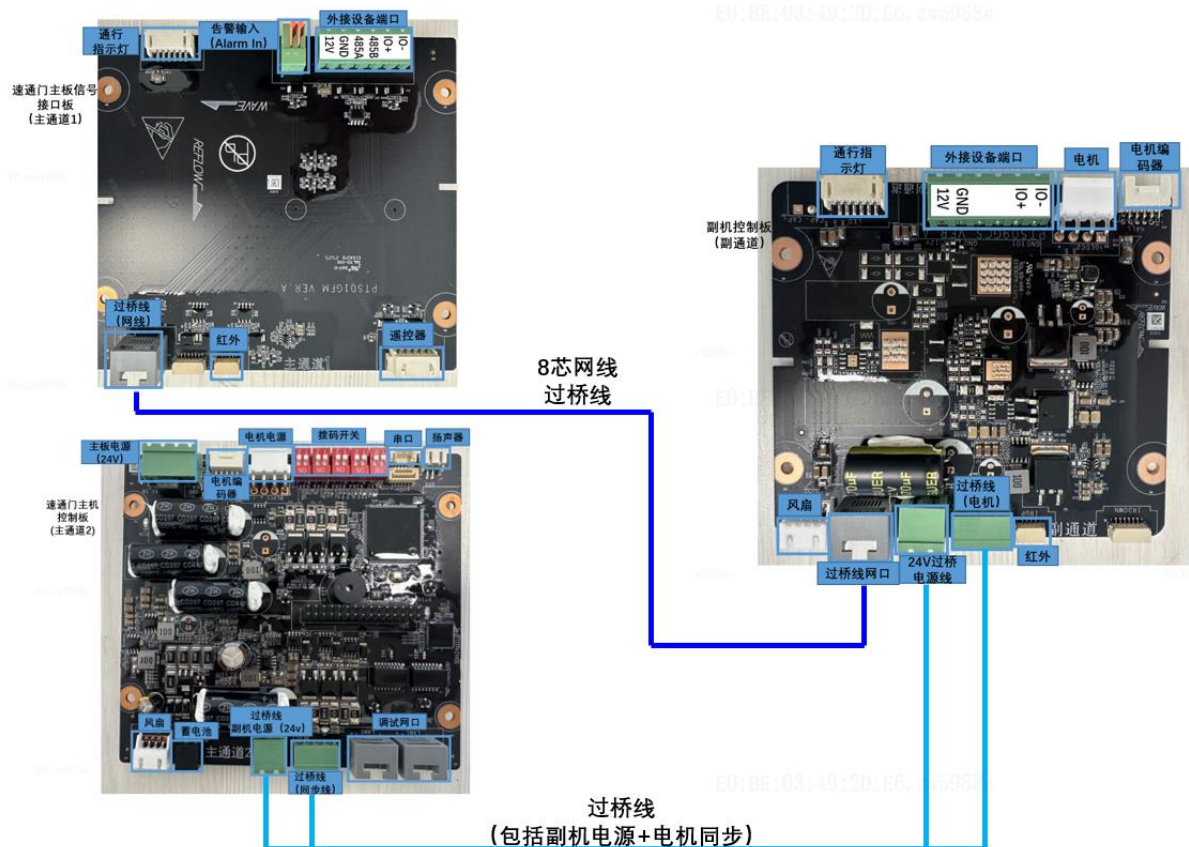
图5-9 过桥线连接
