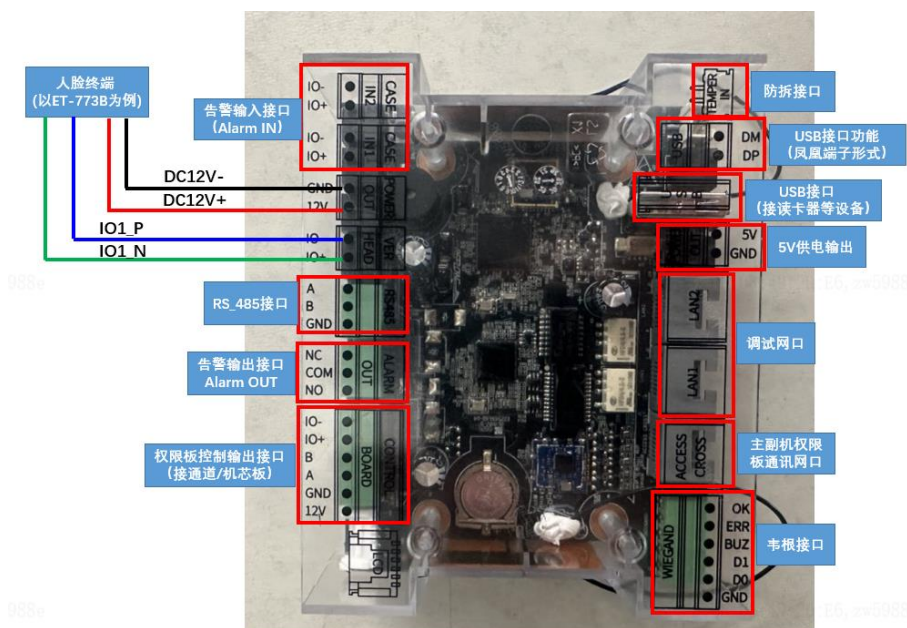
图5-15 核验终端接线图
