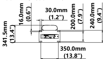
图2-2 尺寸 (单位: mm)
