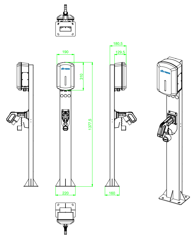
充电桩尺寸图
