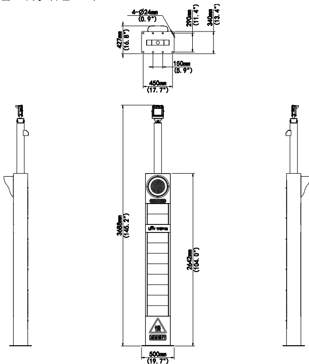
图2-2 尺寸 (单位: mm)
