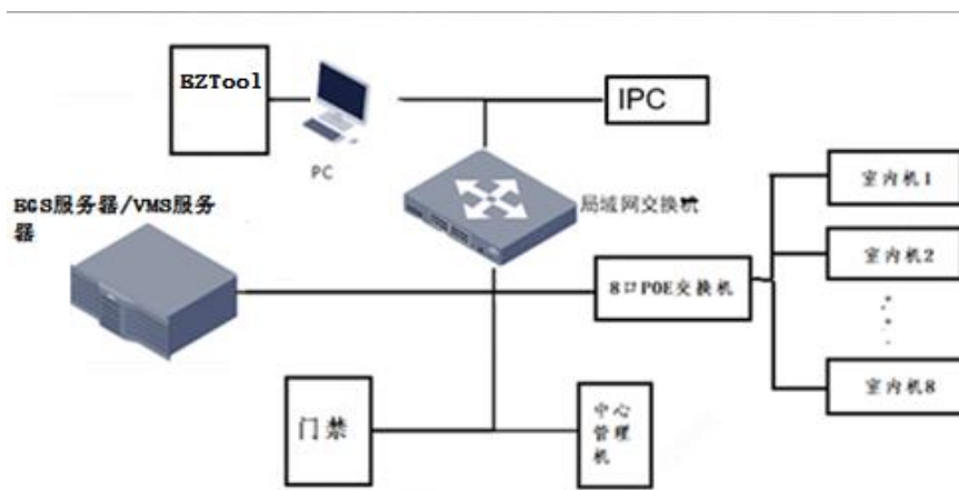
图3-1 设备组网连接图
