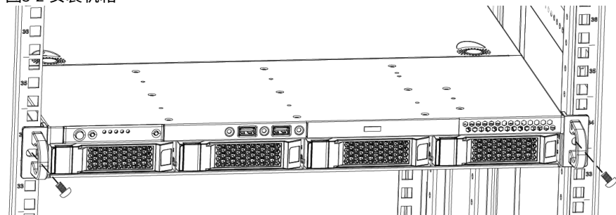
图3-2 安装机箱
