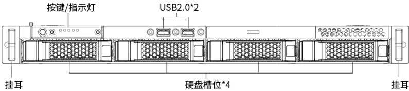
图2-1 前面板结构
