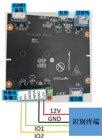
图5-12 智能核验终端接线
