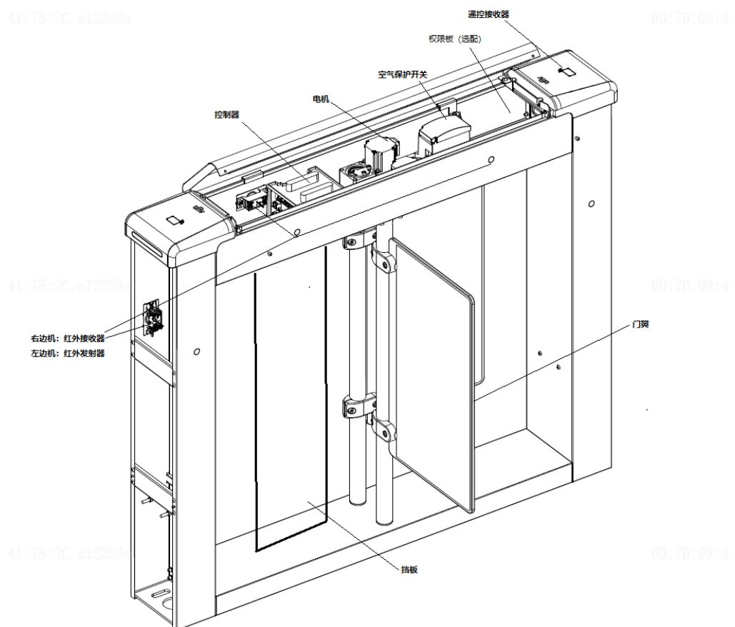
图1-3 图 1-3 整体结构图（以中间边为例）
