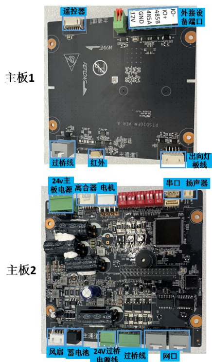
图5-7 主通道板端口介绍
