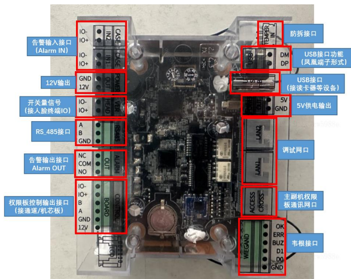
图5-9 权限板端口介绍
