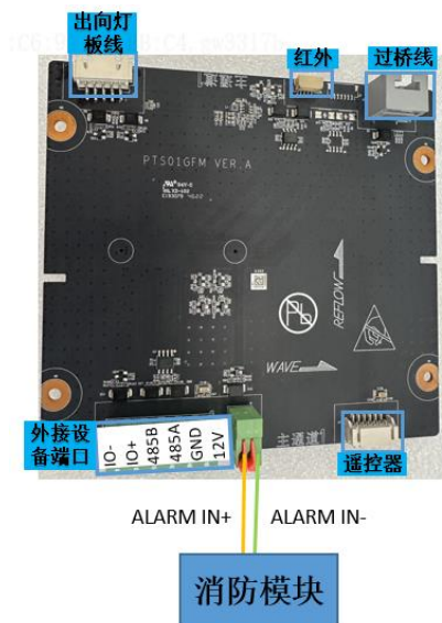
图5-13 消防模块接线
