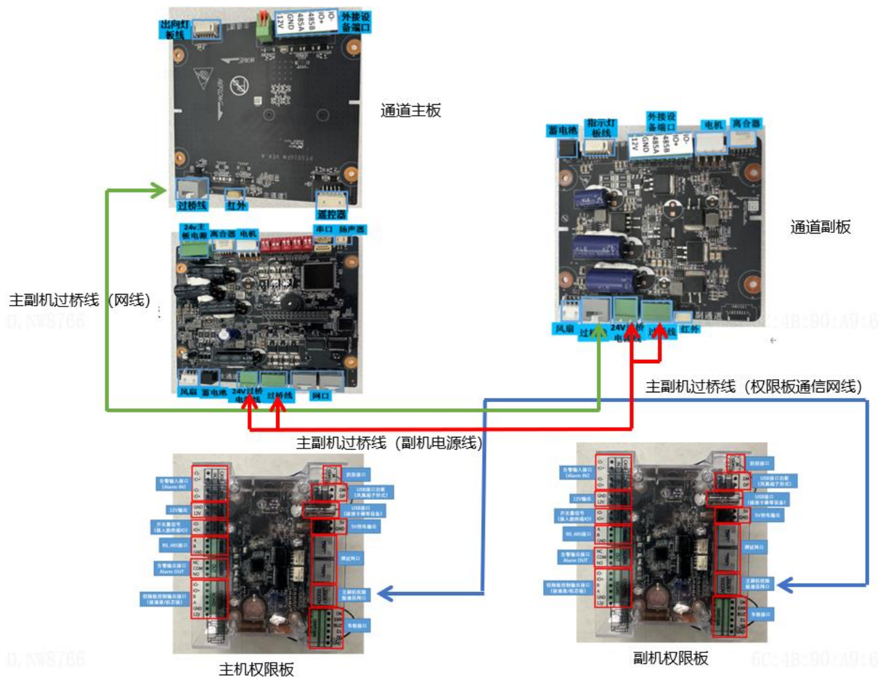
图5-11 过桥线连接
