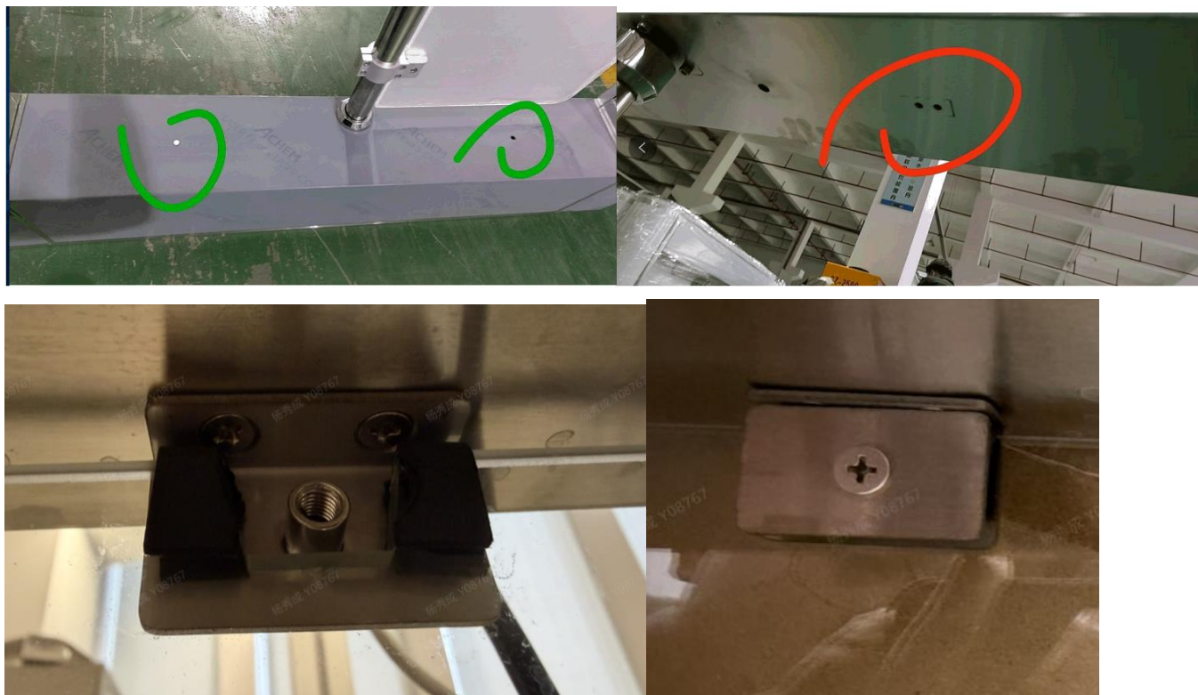
图5-15 侧封板安装
