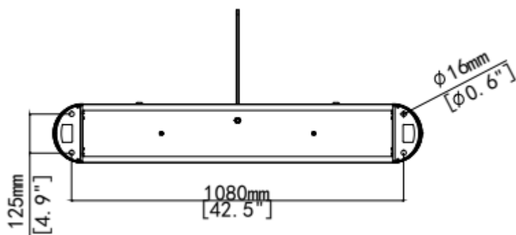
图5-5 FG8201(-ZD)通道安装尺寸图(底视图)
