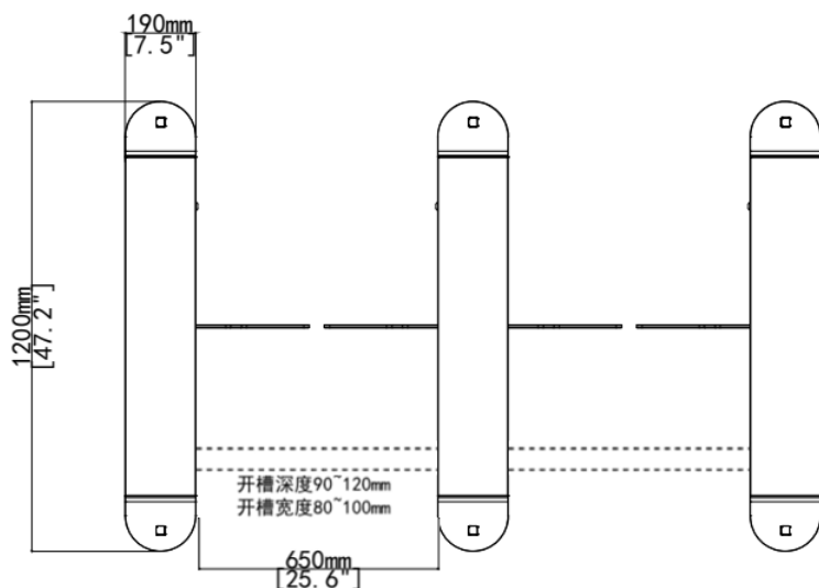
图5-5 FG8201(-ZD)通道安装尺寸图(底视图)
