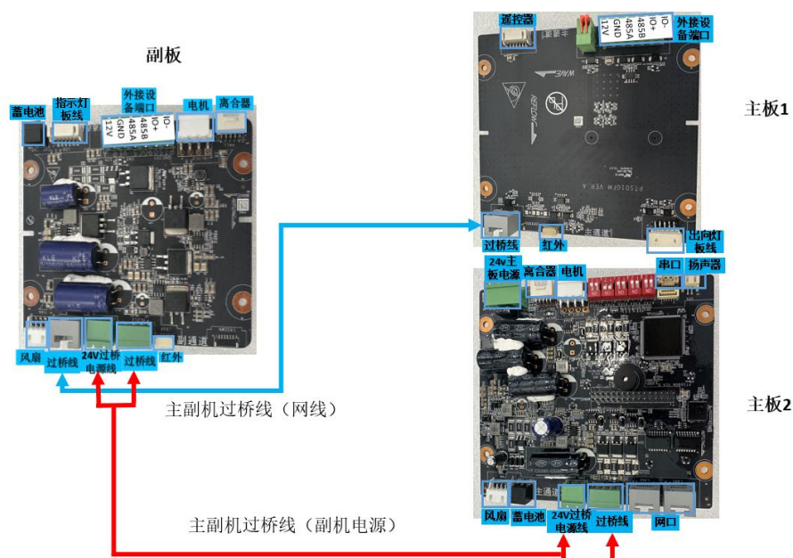
图5-10 过桥线连接
