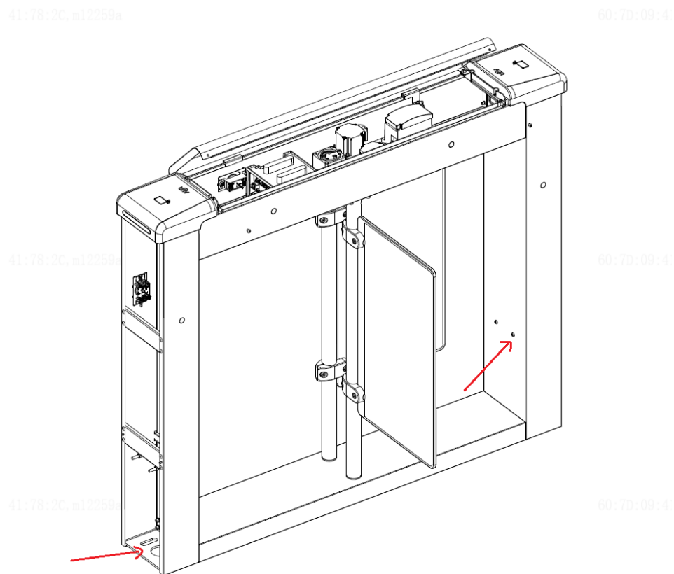
图5-1 打开闸机两侧金属盖板
