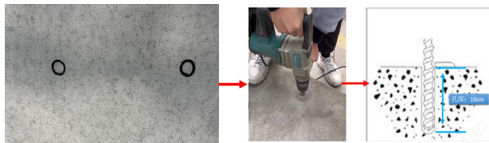
图5-3 标记打孔
