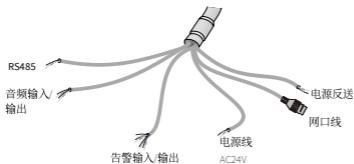
尾线样式二:
