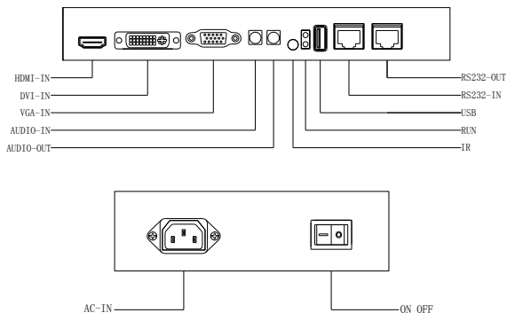
图4-1 产品接口视图
