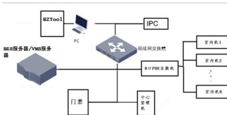
图3-1 设备组网连接图
